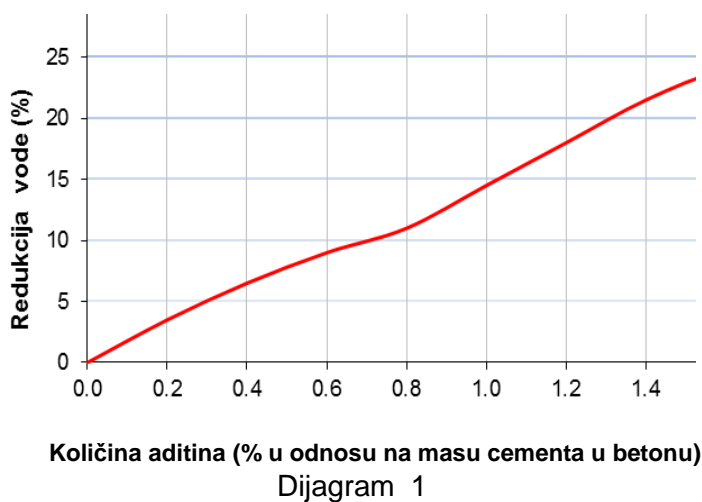
Redukcija vode Saglasno EN 480-1 I EN 934-2, Tabela 3.1
